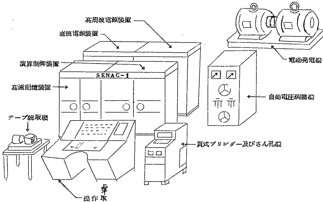
SENAC-1 配置図
